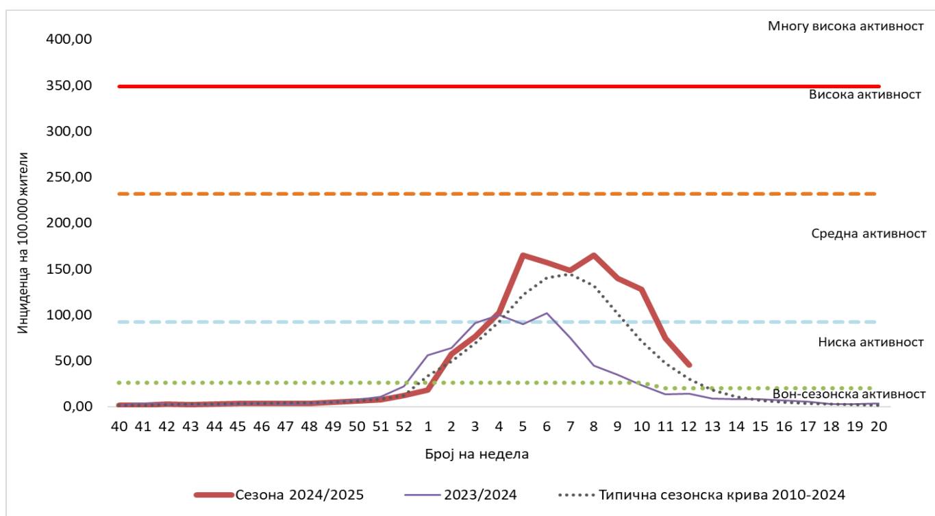
Grafiku 1. Niveli i intensitetit dhe shpërndarja javore e të sëmurëve me grip/ sëmundje të ngjashme me gripin sipas lakores epidemike të pritur 2010-2024, sezoni 2023/2024 dhe sezoni 2024/2025
